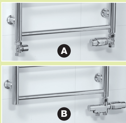
Handdukstork NÄÄS i krom (NKC0860) A + kromat ventilset med termostat (VK11). B + kromad NH-ventil med termostat (NK2). 2
